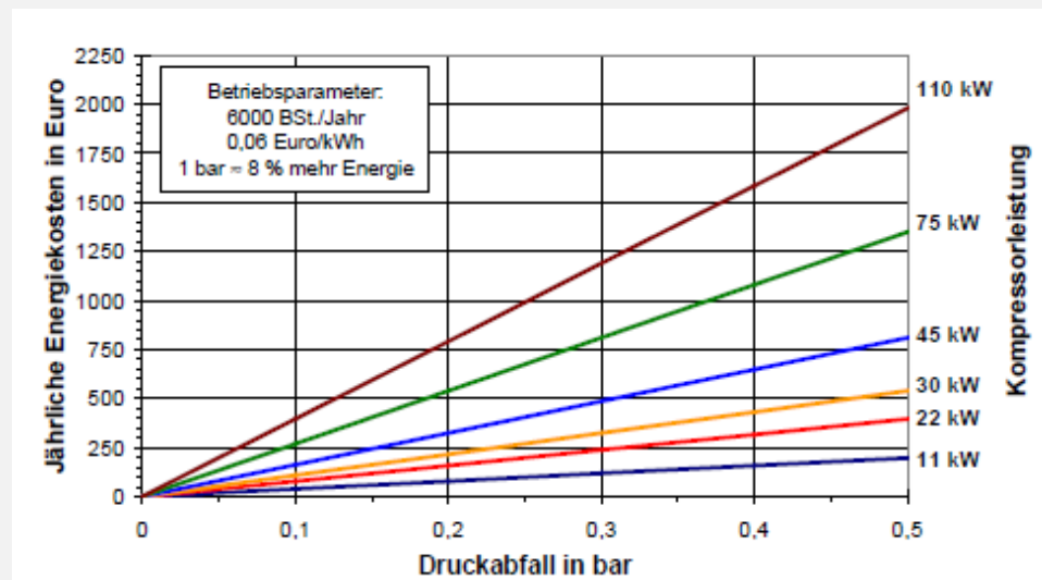
Abbildung 29: Energiekosten Druckluft [23]
